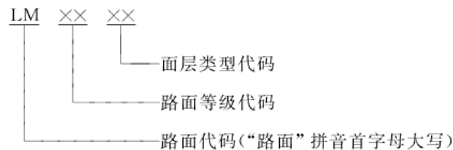
图 1 代码结构
